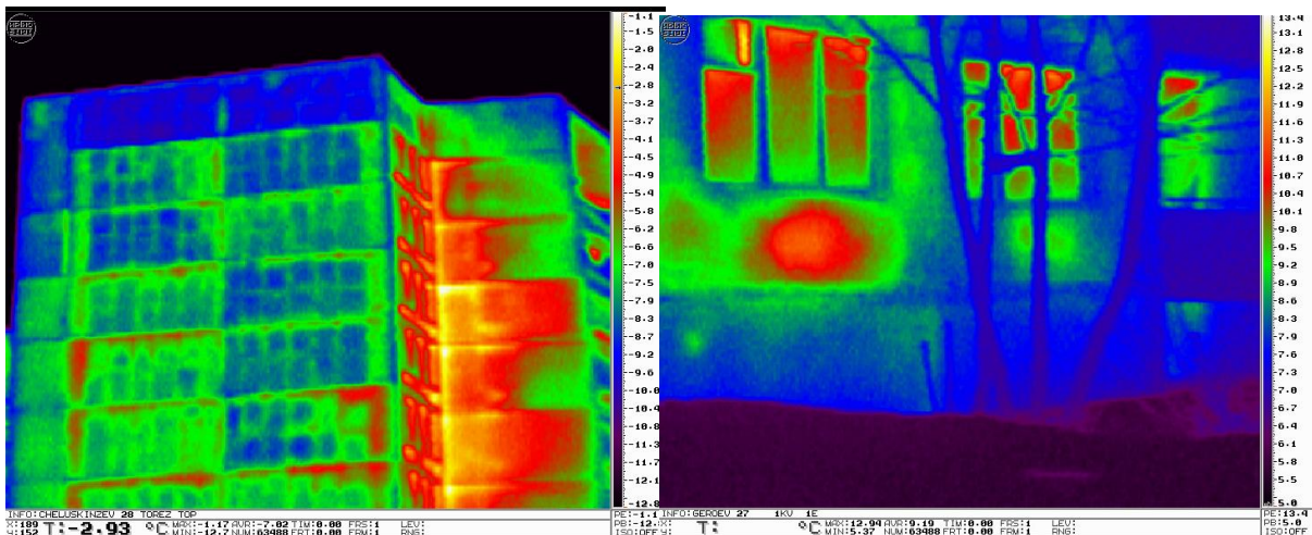
Рис.1 Теплові втрати у житлових будинках
