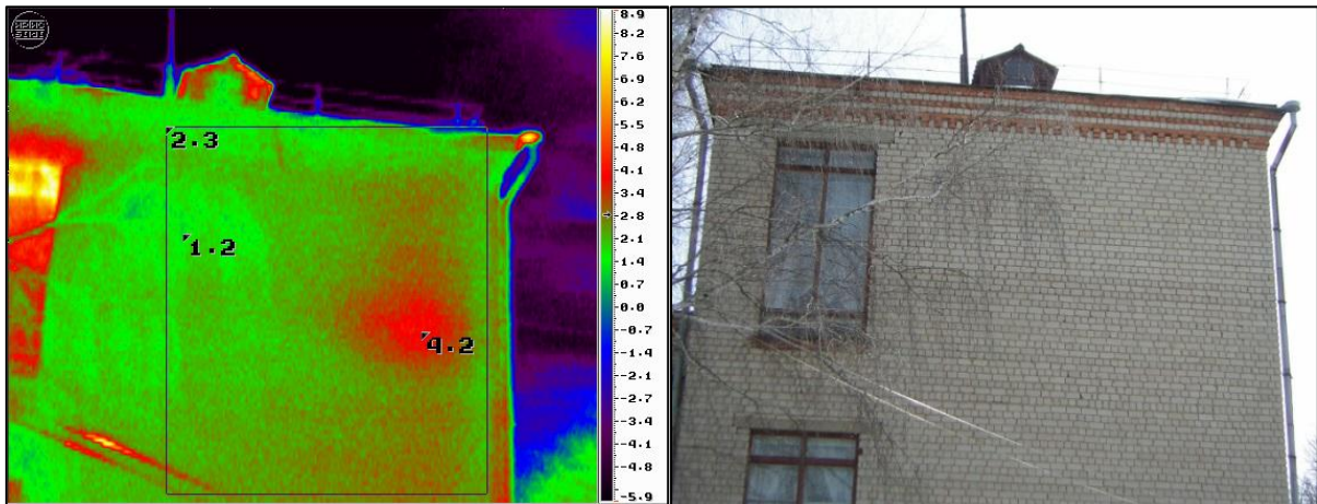
Рис.2 Теплові втрати будівлі спального корпусу школи-інтернату.
